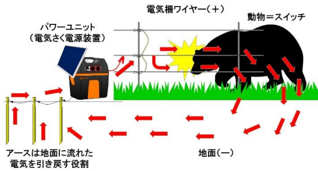
(図1)電気柵の回路
