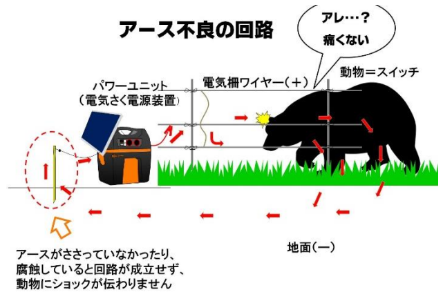
(図2)アース不良の回路では動物にショックが伝わらない
